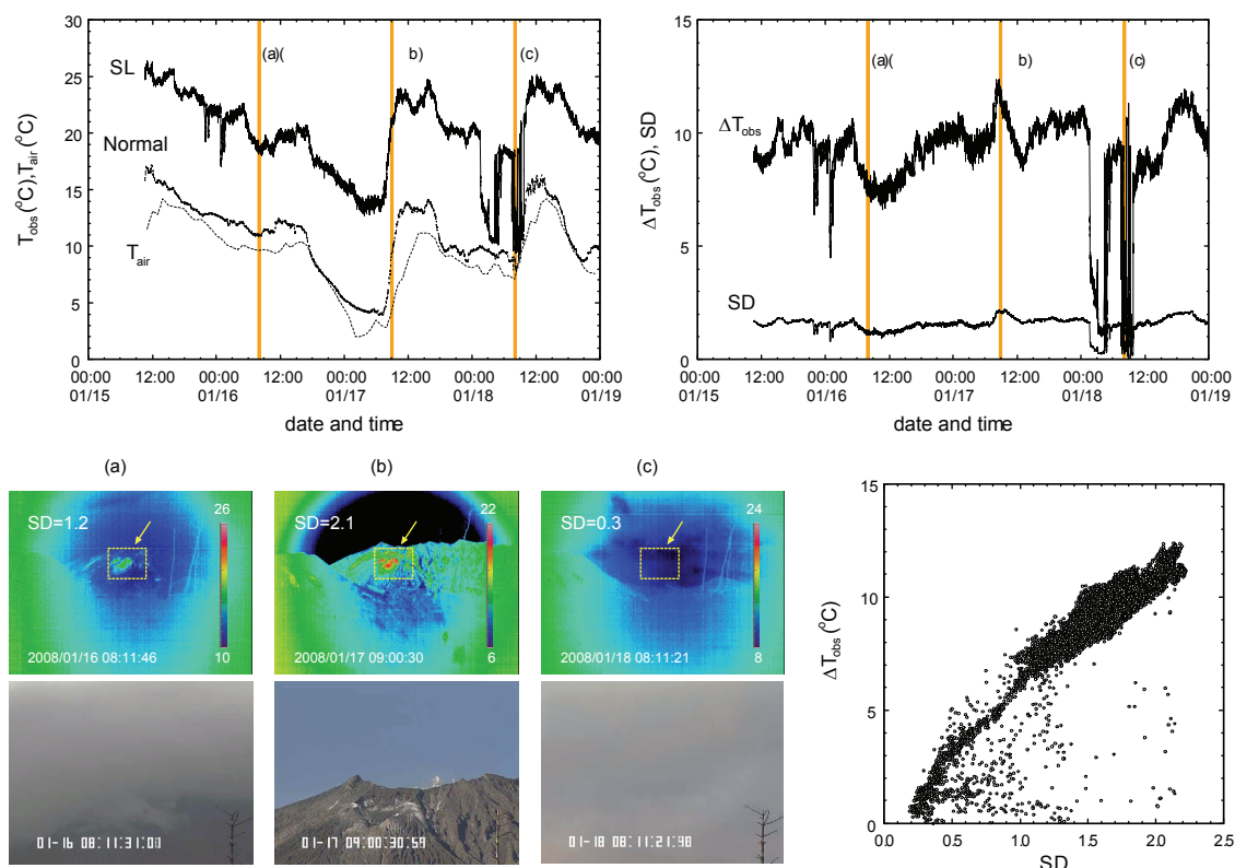
図 6. (上)2008 年 1 月 15 日から 1 月 19 日の観測結果。(左下)時系列グラフ中の(a)~(c)の時刻における・熱赤外画像と可視画像。SD は図中点線で囲まれた矩形領域内 (50×40 ピクセル) で計算した。(右下)およそ 3.5 日分データの \Delta T_{obs} と SD の関係。正の相関が認められる。
