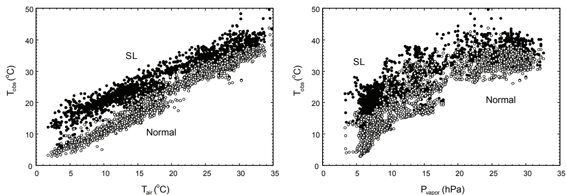
図 5. 鹿児島市における大気温度 T_{\text{air}} (左), 水蒸気圧 P_{\text{vapor}} (右)と, SL(●), Normal(○)で観測された最高温度, 平均温度との関係(2007 年 8 月 9 日から 2008 年 1 月 17 日)。
