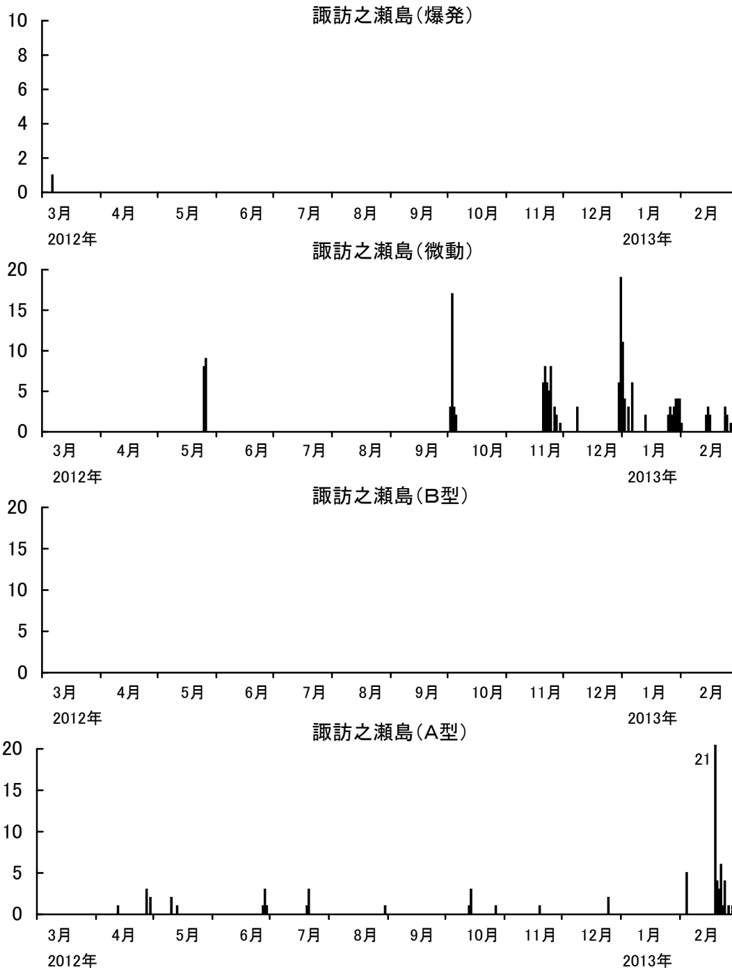
諏訪之瀬島における火山性地震の日別発生回数 (2013年2月28日まで)
