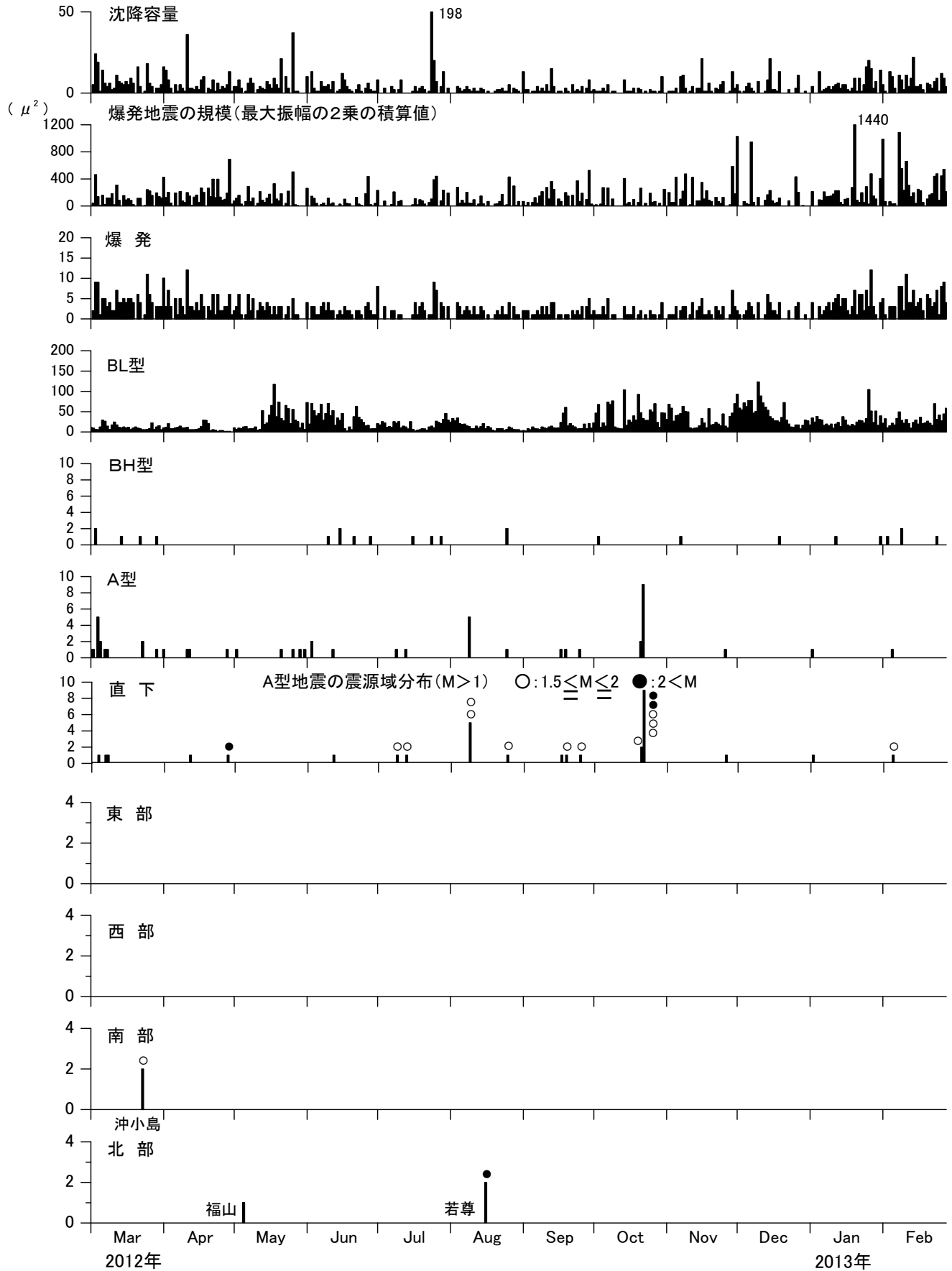
火山性地震の日別発生回数(2013.2.28まで)
