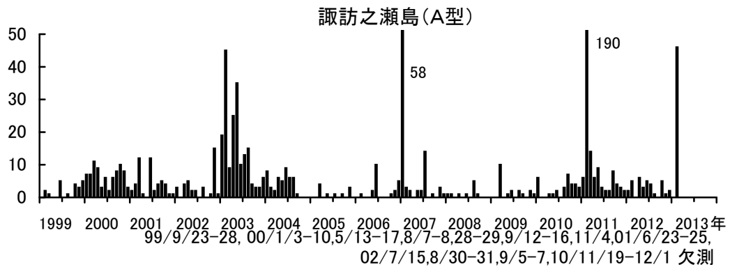
諏訪之瀬島における火山性地震の月別発生回数 (2013年2月28日まで)
