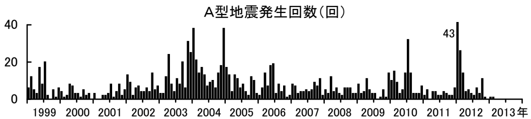
桜島における火山性地震の月別発生回数と降下火山灰量 (2013年2月28日まで)
