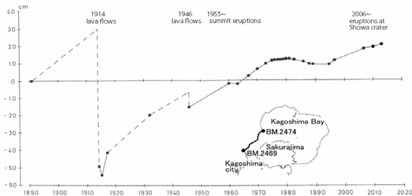
BM. 2469を基準としたBM. 2474の比高の経年変化 (最新データ : 2012年11月)
