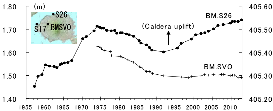
BM. S17を基準としたBM. S26およびBMSVOの比高の経年変化 (最新データ : 2012年12月)
