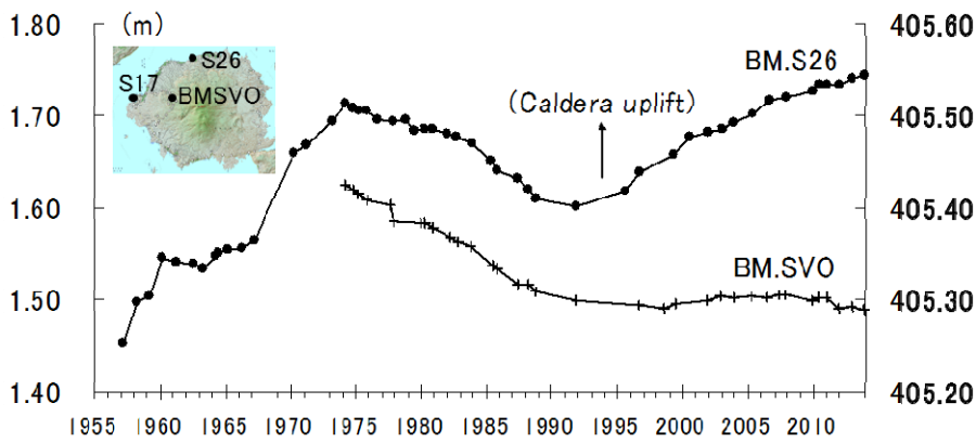
BM. S17を基準としたBM. S26およびBMSVOの比高の経年変化 (最新データ: 2013年11月)
