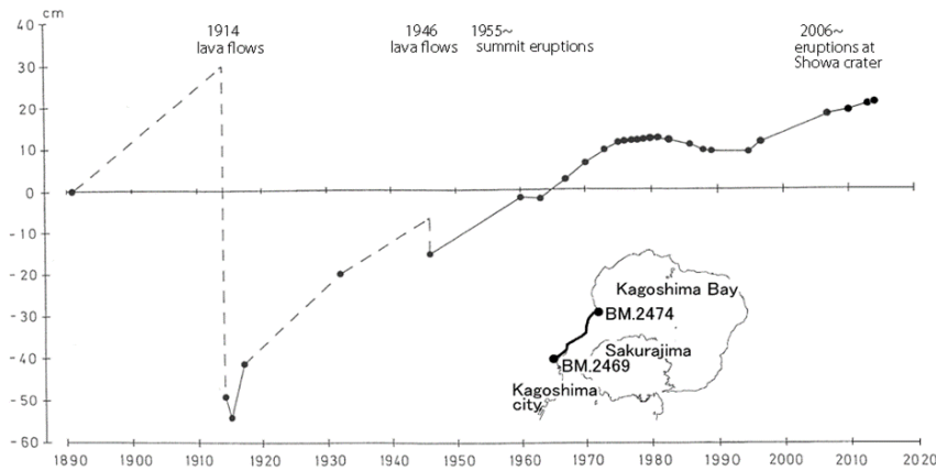
BM. 2469を基準としたBM. 2474の比高の経年変化 (最新データ: 2013年11月)
