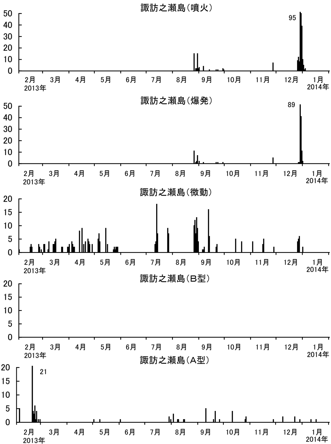
諏訪之瀬島における火山性地震の日別発生回数 (2014年1月31日まで)
