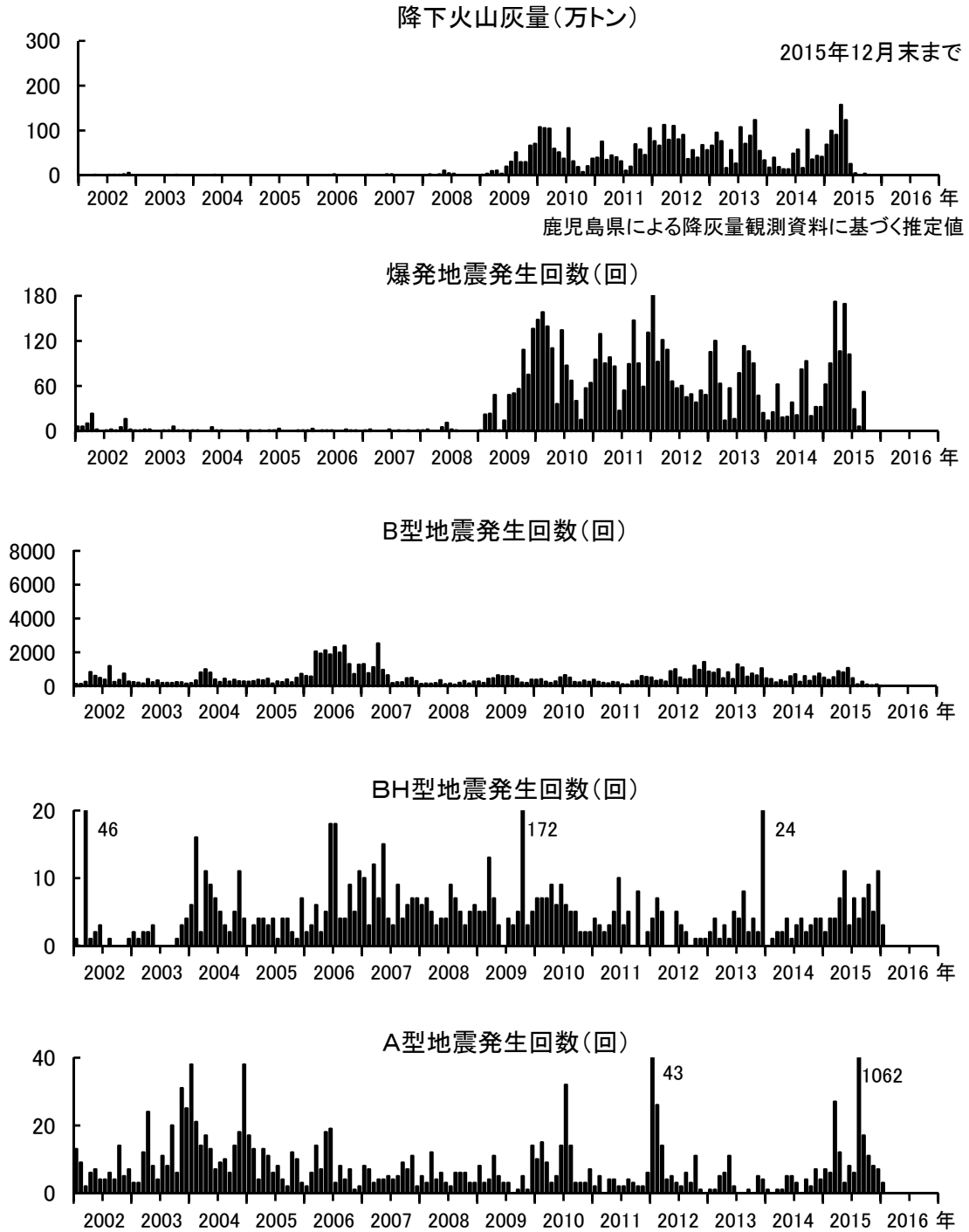
桜島における火山性地震の月別発生回数と降下火山灰量 (2016年1月15日まで)
